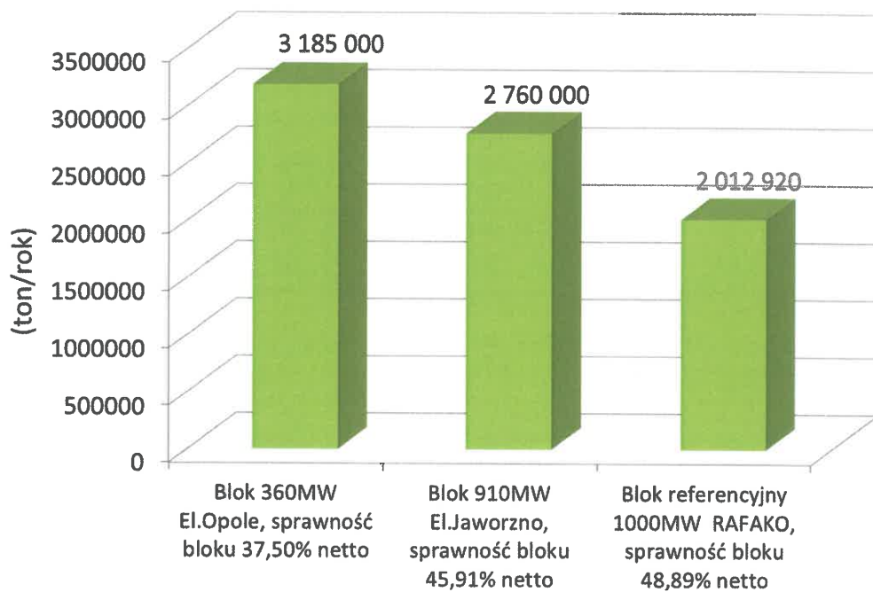
Rys. nr 10.8. Roczne zapotrzebowanie na węgiel
